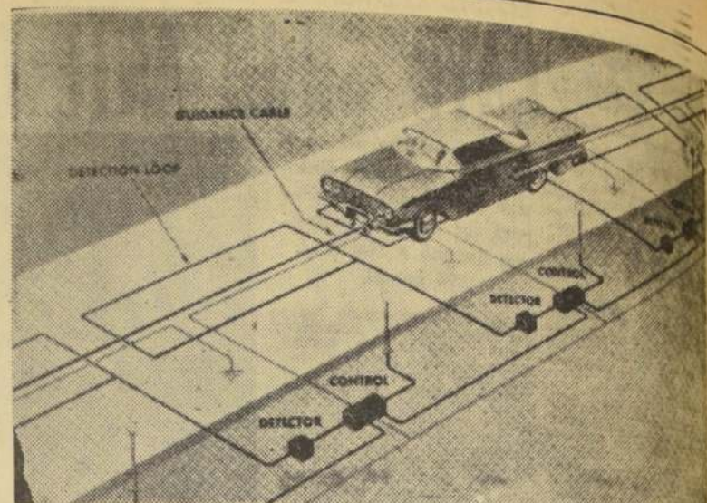
Dibujo esquemático de la carretera electrónica desarrollada por R. C. A. Se pueden observar los cables colocados bajo el pavimento. En este grabado, el circuito de control de la huella luminosa detrás del coche que avanza, para advertir a los otros vehículos de su presencia.
