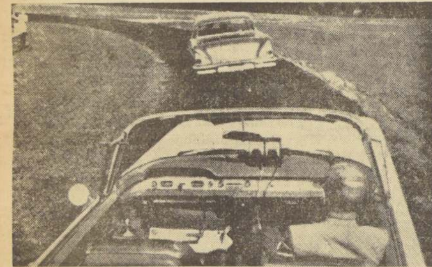
El coche avanza en el Centro de Investigación David Sarnoff, en Princeton. Este coche sigue automáticamente la prueba circular y se detiene para evitar una colisión con el coche de prueba que va adelante. Los dos instrumentos colocados en el parabrisas indican la velocidad y la distancia del coche que va adelante, mientras esta información se recibe directamente desde el camino por los instrumentos electrónicos que lleva el coche.
