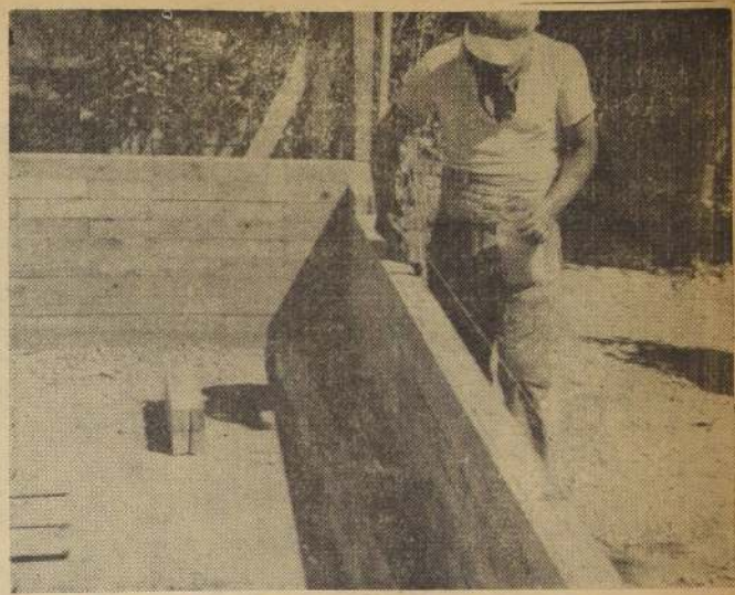
En el sistema de bloques de madera no se necesita ser obrero constructor ni especializado. El grabado explica cómo se colocan. Este propietario pone sobre la hilada de bloques un brochazo de cola plástica, con catalizador.
