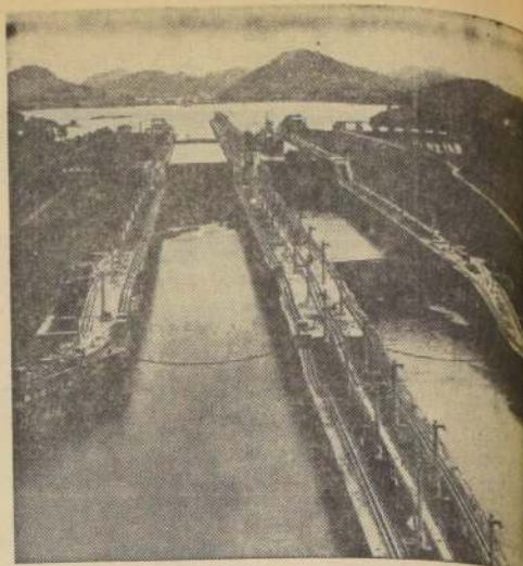
ESLUSA DE MIRAFLORES. SALIDA AL OCEANO PACIFICO EL CANAL DE PANAMA.
