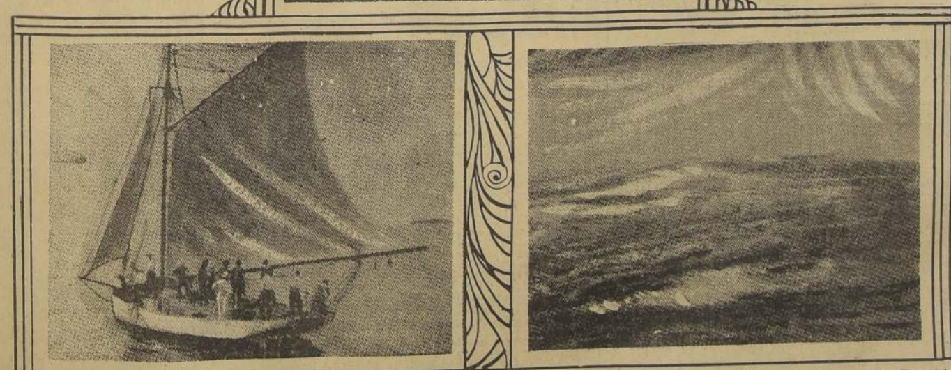
1.— La Isla Halcón, en el Pacífico Sud, que dos veces ha desaparecido a causa de los tremendos cataclismos que se han producido en ella. Esta isla es de origen volcánico. Actualmente, el volcán que hay en su parte central está en actividad; arroja grandes cantidades de lava, humo, emanaciones venenosas, etc. El agua está corroyendo sus costas y es muy posible que pronto vuelva a desaparecer.— 2.— La partida de expedicionarios, saliendo del puerto de Nukualofa, capital del grupo de las islas Tonga, a bordo del cutter "Fetunaho", con rumbo hacia la isla desaparecida.— 3.— El lago hirviente, situado en el cráter del pequeño volcán está rodeado por altas murallas de cenizas y grandes moles de azufre cristalizado. Espesas nubes de vapor de agua cubren constantemente la superficie de este extraño lago.
