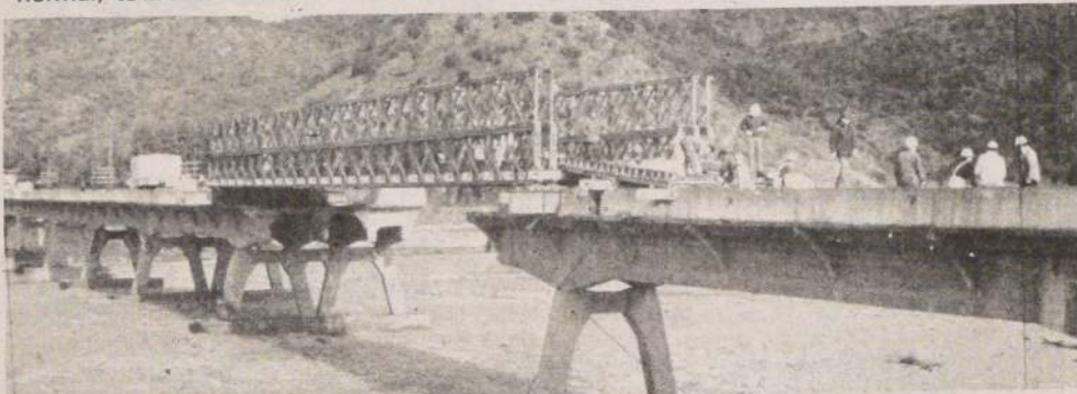
Reforzado con un puente mecano tipo Bailey, la próxima semana el viaducto sobre el Tinguiririca estará habilitado para el tránsito vehicular sin límite de peso.
