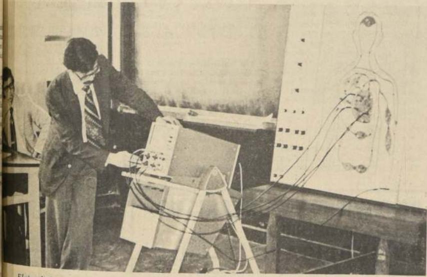
El simulador cardiovascular de la Universidad Santa María está hecho de equipos electrónicos con componentes de alta tecnología. En la foto, opera el simulador electrónico el profesor Héctor Ibáñez, y observa Daniel Rodríguez.
