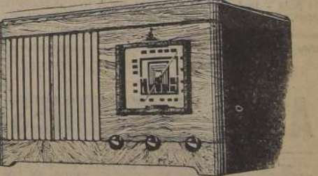
Modelo 331-X 6 tubos con rendimiento de 8. Circuito superheterodino. Corriente Universal. Gabinete acústico Parlante de 8" con gran calidad de tono.
