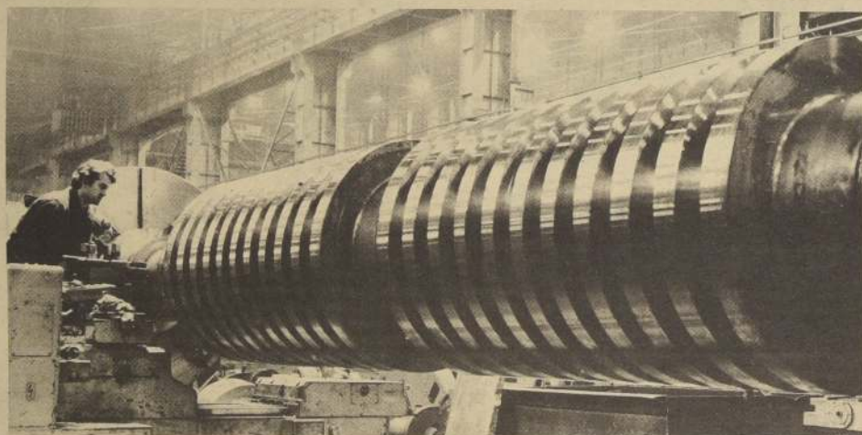
Labrado del rotor para una turbina de 500 mil KV en la fábrica Talicheski de Leningrado.
