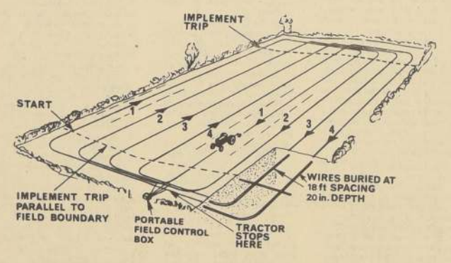
Diagrama ilustrativo del sencillo sistema de "red de cables" para el tractor sin conductor. Si se realiza un trabajo de drenaje la red puede ser sepultada a mayor profundidad, por un costo ligeramente superior. 1) Punto de partida; 2) Límite de recorrido del implemento; 3) Cables sepultados a intervalos de 5,49 metros y 0,50 metros de profundidad; 4) Punto de detención del tractor; 5) Caja portátil de control de campo; 6) El límite de recorrido del implemento es paralelo al límite del campo.
