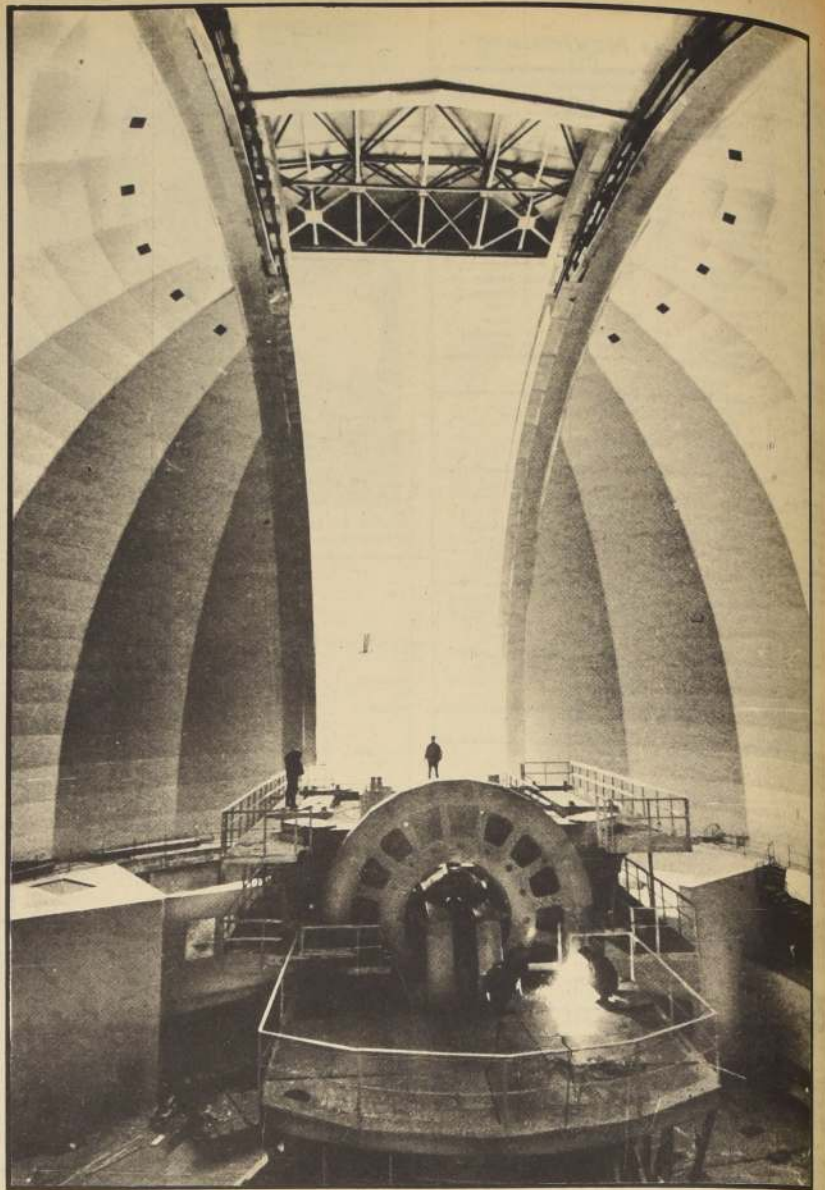
Esta es la rendija para el telescopio que cerrarán las cortinas de lavsán de 1500 metros cuadrados.
