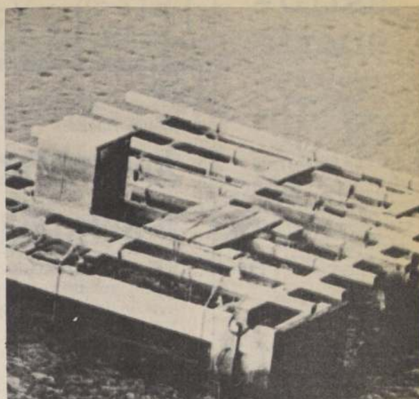
Balsa experimental en el estuario del río Queule: un laboratorio flotante en busca del conocimiento biológico de choros y choritos.
