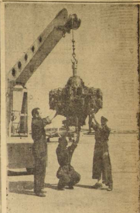
Expertos mecánicos de LAN-CHILE practican los últimos ajustes a un motor de los aviones de esa Empresa, antes de ser instalado en el potente y moderno Banco de Frusba de Motores, en donde se controla rigurosamente su funcionamiento, con precisión y exactitud idénticas a como funciona colocado en el aparato a que pertenece.
