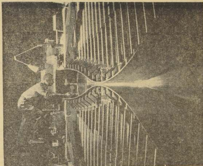
Un experimentador norteamericano ensaya el motor de un gran túnel de viento, supersónico, de modelo de una nueva proyectil teleguiado de abertura variable.
