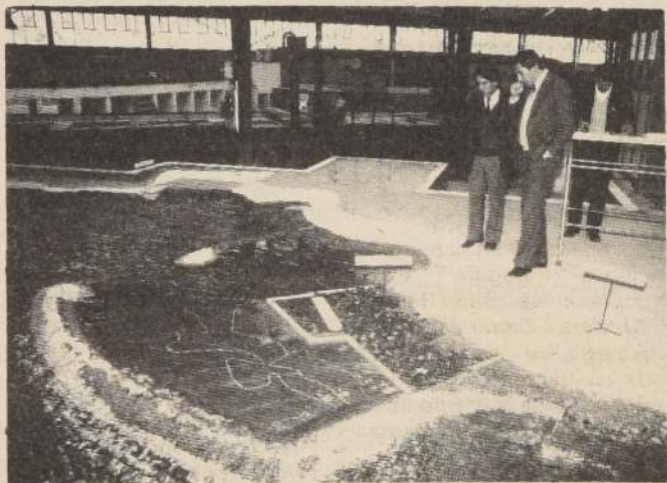
Los ingenieros del Instituto Nacional de Hidráulica prueban con maquetas y simuladores, en su laboratorio de Peñaflor, los materiales más indicados para la construcción del puerto.
