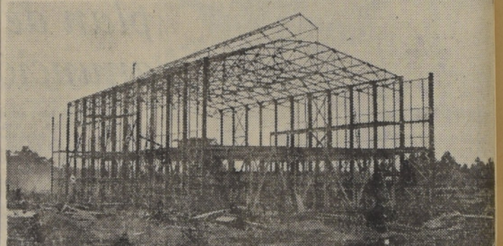
ESTRUCTURAS METALICAS.— Las fotografías no son recientes. Los trabajos están aun mucho más avanzados. La planta de azúcar quedará terminada en marzo y se inaugurará solemnemente el primero de abril próximo. 700 operarios trabajan simultáneamente en levantar las estructuras de los edificios y en instalar las maquinarias y elementos de trabajo que, en un 90 por ciento están ya en el país.
