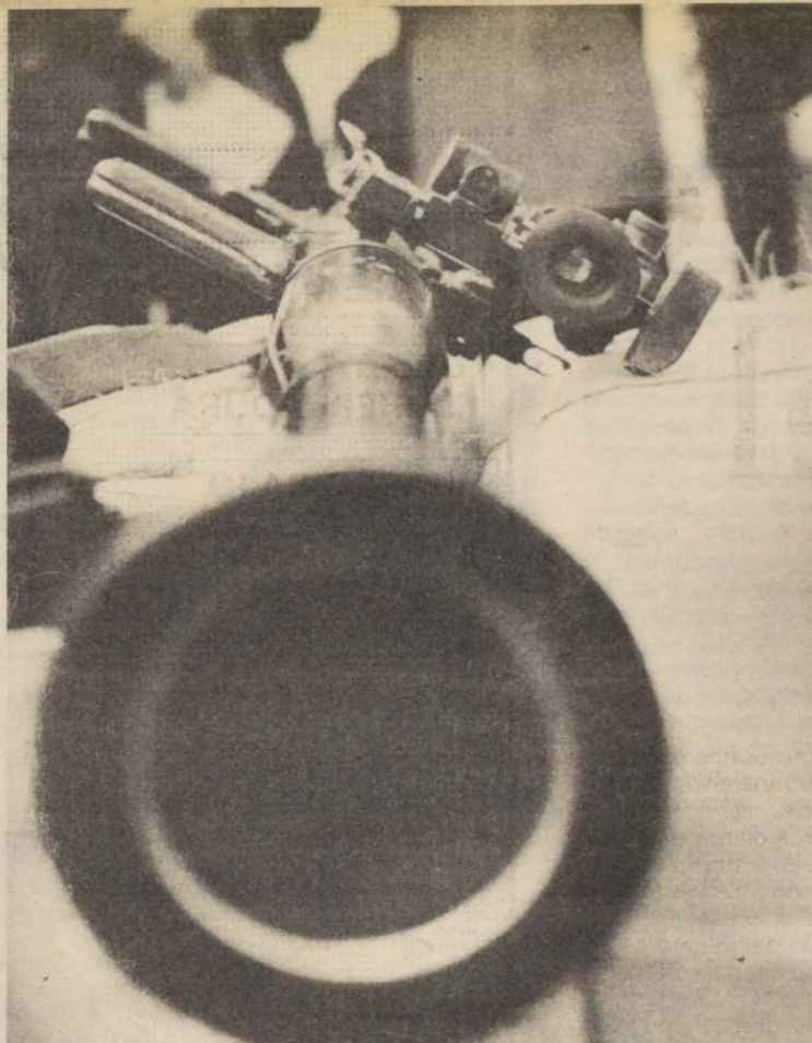
Un lanzacohete RPG-7V antiblindaje, el más moderno en su género en uso en todo el mundo. Es fabricado por la Unión Soviética.
