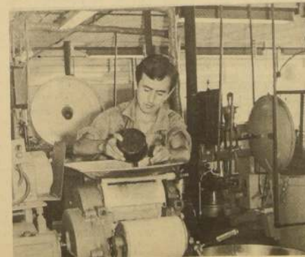
En esta maquina separadora de pulpa, espina y pellejos, comienza la transformación del pescado en un polvo blanco, inodoro e insípido, que no es otra cosa que un rico concentrado proteico, puro, indispensable para la alimentación de hombres y animales.
