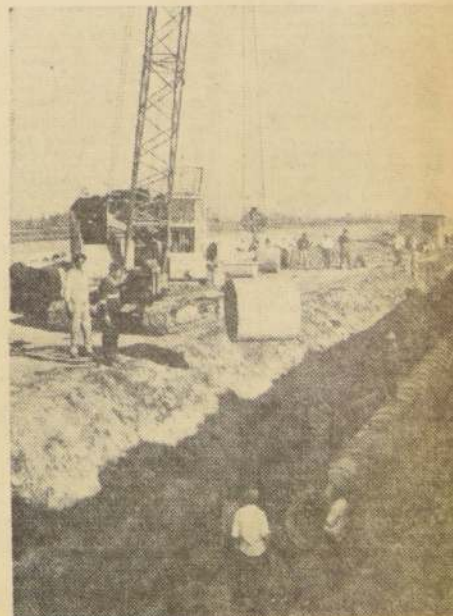
Tubos VIBROCRET en Pudahuel. Obreros proceden a la colocación de las tuberías que servirán para la captación de aguas y drenajes de toda el área del Aeródromo de Pudahuel.
