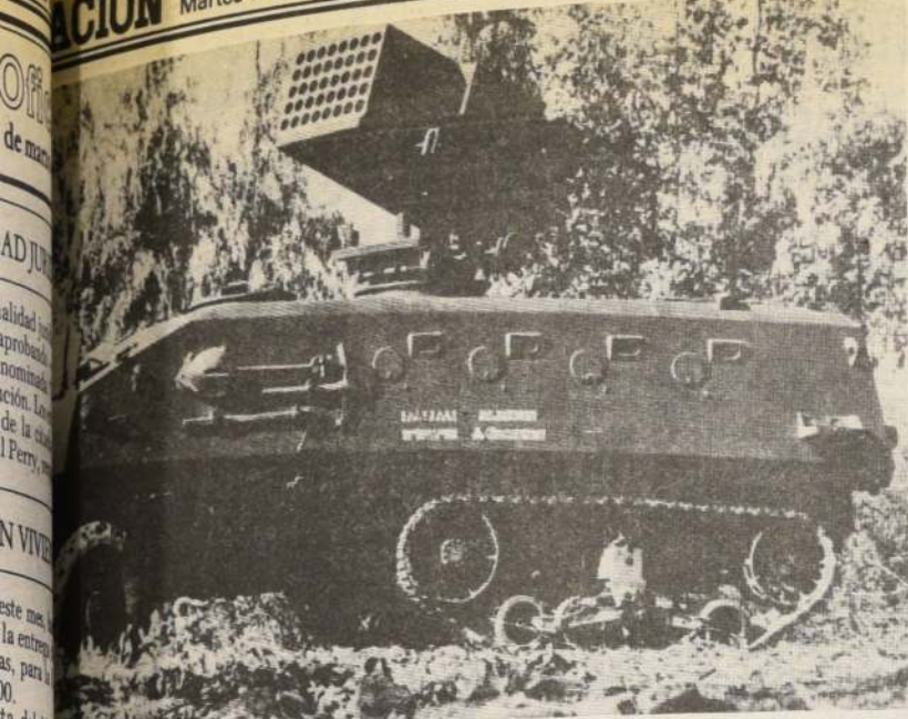
El múltiple semioruga BMS-1 "Alacrán", fabricado por la industria chilena en su división de defensa. Es de uso múltiple y puede ser equipada con armamento antitanque, antiaéreo o antipersonal.
