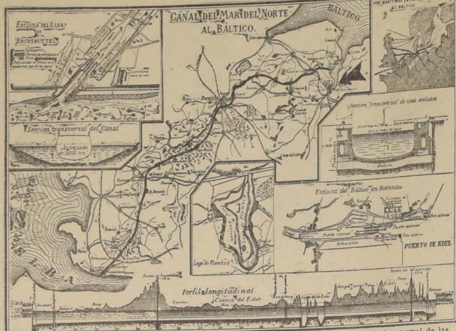
Plano del Canal de Kiel.— Perfil longitudinal y sección transversal del mismo.— Plano y sección transversal de las esclusas.— Plano del lago de Flehmud y vías marítimas entre el mar del Norte y el Báltico
