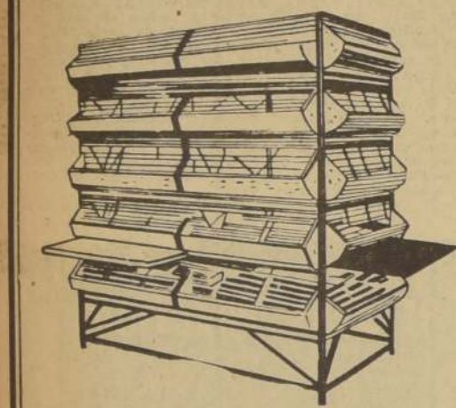
BATERIA DE CRIANZA, TIPO BUCKEY, PARA 1.000 POLLITOS DE 1 DIA
