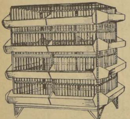
BATERIA DE RECRÍA, TIPO BUCKEY, PARA 400 POLLOS HASTA LAS 12 SEMANAS
