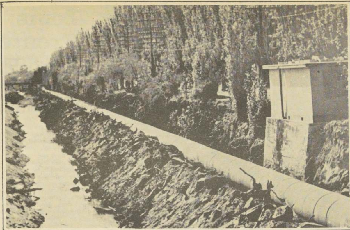
EL 15 de Octubre será entregado el colector industrial "El Salto", para terminar con los malos olores del estero de Viña. En la foto, un tramo de la tubería de 6,5 kilómetros de largo que fue necesario colocar a un costado del estero.
