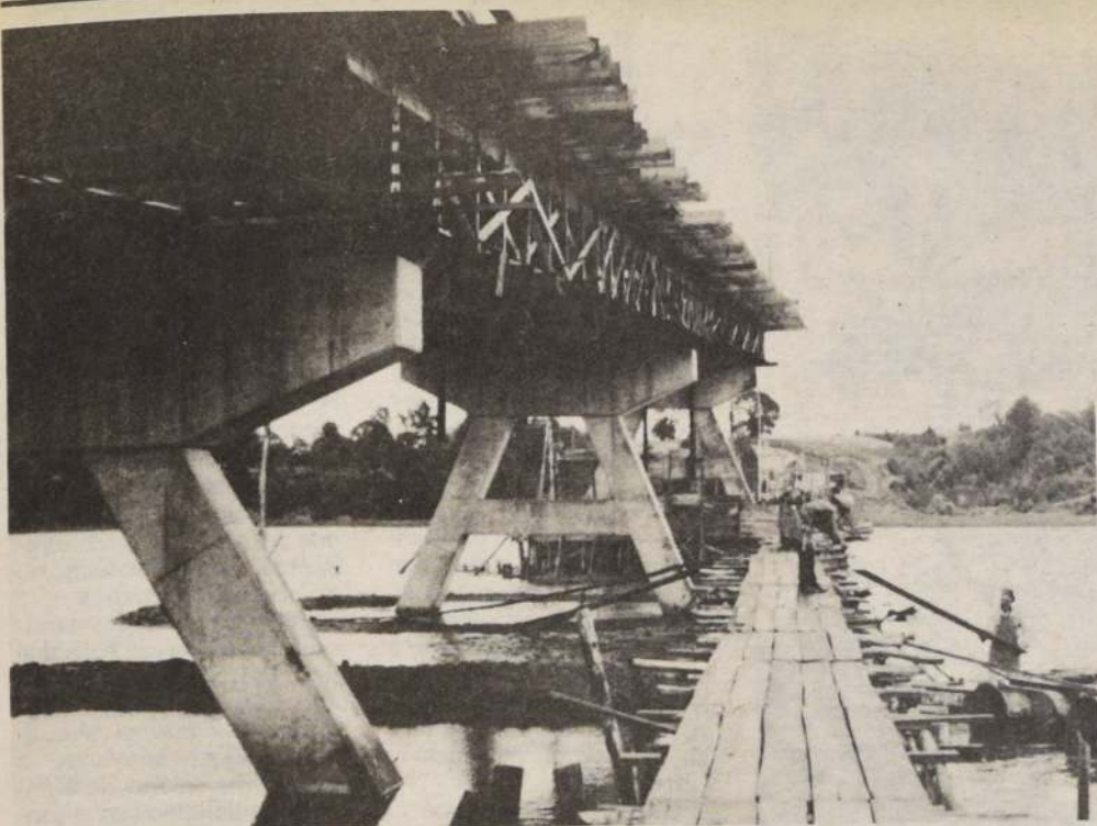
Un notable avance se ha logrado en la construcción del puente Cruces, sobre el río Valdivia, que unirá esta ciudad con Niebla. En la foto, el aspecto que actualmente muestra esta obra.
