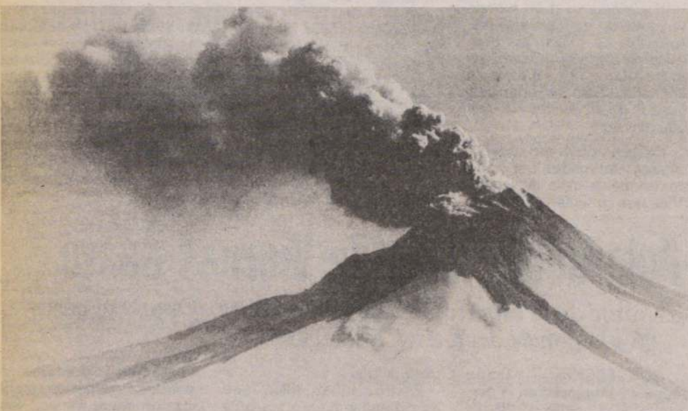
ERUPCION VOLCANICA, una espesa nube de humo y cenizas se eleva del volcán Augustine. Las erupciones del volcán han hecho caer ceniza sobre Anchorage, Estados Unidos, y una extensa zona cubierta por las nieves. El humo hizo detener el tráfico aéreo en la zona y las autoridades sanitarias advirtieron a los habitantes del lugar que se mantuvieran en el interior de sus casas. (Reuter).
