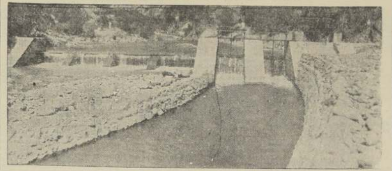
Toma en las obras de regadío de Colina.
