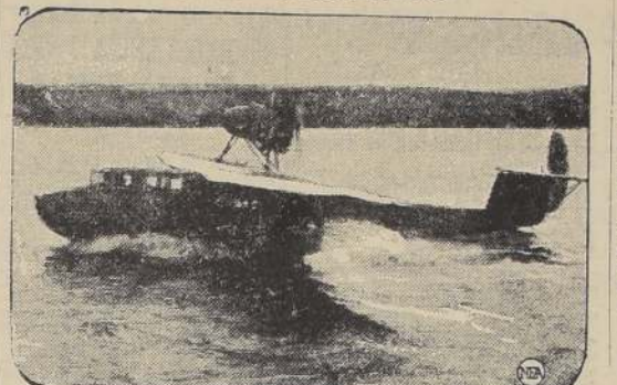
Este gigantesco hidropuerto, al cual la fotografía muestra desfilando por el agua antes de despegar en el río Hackensack, Nueva Jersey, es la aeronave "misterio" producida ultimamente por Fokker para la aviación comercial. El casco de la gondola fue construido en Holanda y, según se dice, se caracteriza por la cantidad de novedades que ofrece en cuanto a diseño y construcción.
