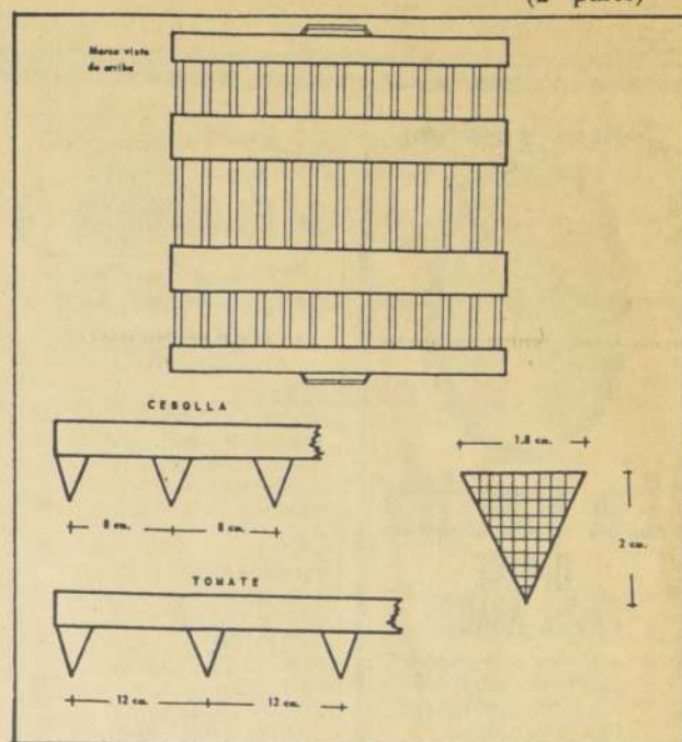
Marco rayador para la siembra de almácigos en líneas de hortalizas.
