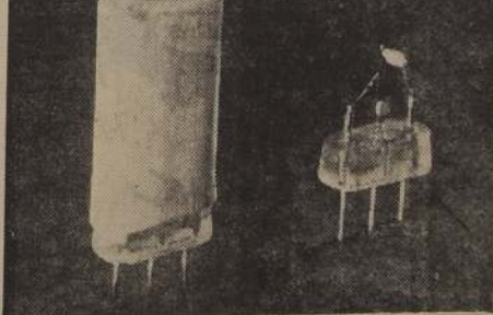
A LA IZQUIERDA, aspecto externo de un Transistor. A la derecha detalle interno, con sus tres alambres, placa y trozo de germanio, que son posteriormente recubiertos por una tapa de plástico. La punta del lápiz permite apreciar sus escasas dimensiones, no mayores que un grano de maíz.
