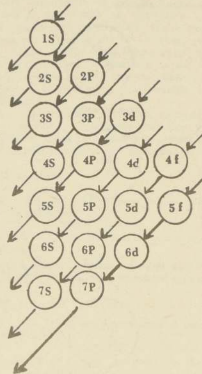
Orden en que se llenan los orbitales atómicos
