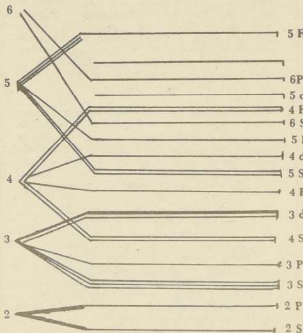
Orden en que se llenan los orbitales atómicos
