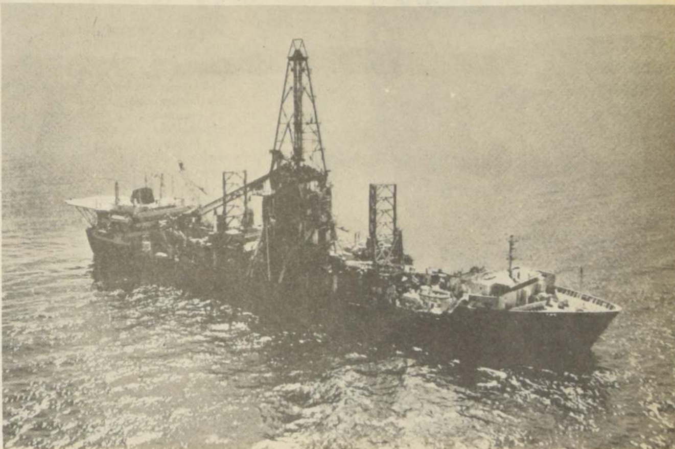
El barco minero debe estar cuatro años inmóvil, sin desplazarse su eje central. De él sale una tubería de unos 4.000 metros, que lo conecta con el colector que rastrea el fondo marino. Su inmovilidad se controla vía satélite o a través de boyas sónicas, cuyas señales son captadas por un computador
