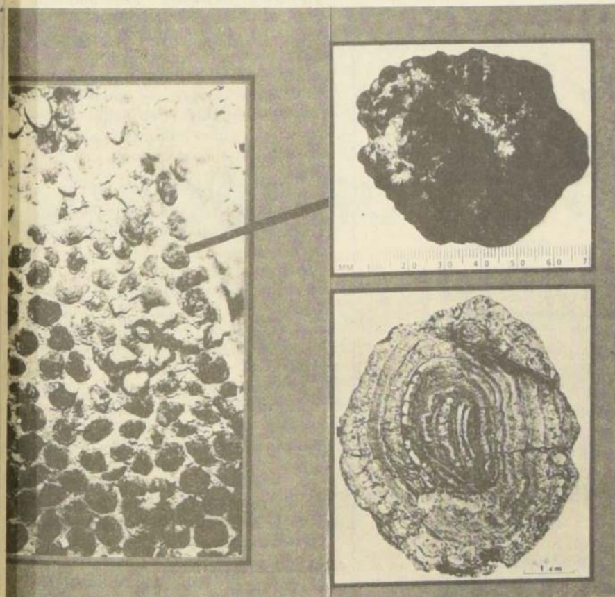
Los nódulos de manganeso representan las mayores reservas de cobre, níquel, cobalto y manganeso conocidas hasta hoy en el planeta.
