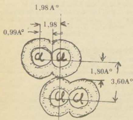
2 moléculas de cloro ( \text{Cl}_2 )
