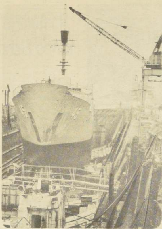
El buque Piloto Pardo en faenas de reparación en el dique menor de ASMAR
