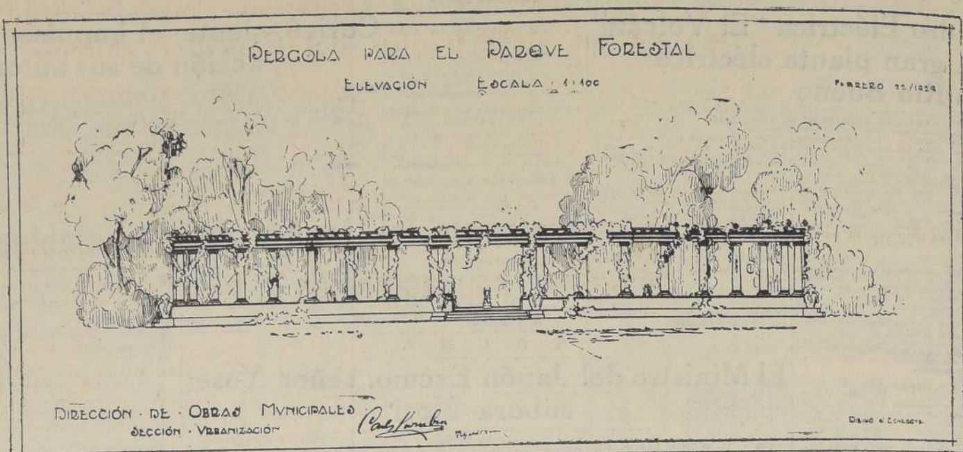
Planos de la nueva pérgola que se construirá en breve cerca de la Fuente Alemana.
