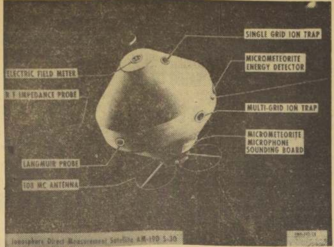
Este es el diagrama del satélite de medición directa de la ionosfera, que fue lanzado exitosamente por Estados Unidos. El equipo ha sido diseñado y construido por el Centro Goddard de Vuelos Espaciales y cuenta con los ocho equipos indicados en el grabado.— (FOTONASA PARA LA UPI).
