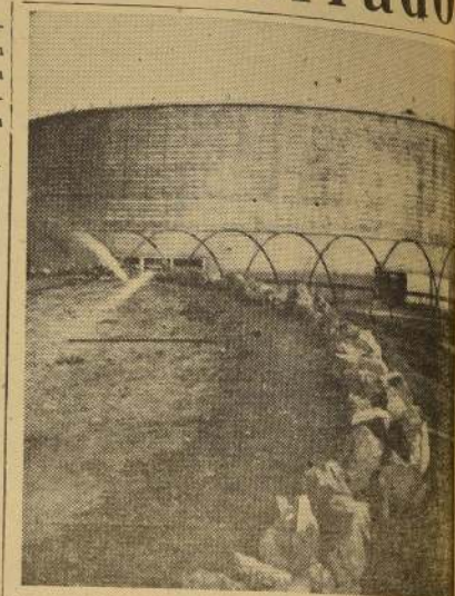
UN CILINDRO. — Es la forma que tiene el local que sirvió para la Exposición Nacional de la Producción Uruguaya. El techo es colgante y para sostenerse no necesita de columna alguna. Es una malla de cables de acero que penden de un arco central. El local tiene una capacidad de 25 mil personas.
