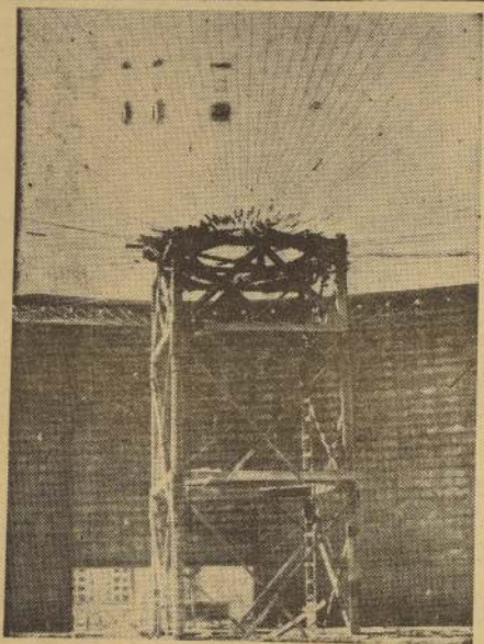
EN PLENA CONSTRUCCION. — El grabado muestra la torre que sirvió para elevar el arco central y por la cual se colocaron los cables de acero del "techo colgante" del local de la Exposición Nacional de la Producción del Uruguay. Esta misma experiencia se podría aplicar en la construcción del estadio cerrado de Santiago.
