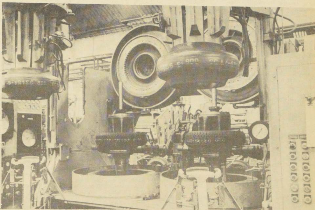
NEUMATICOS radiales G-800 salen de la prensa de vulcanización de la fábrica Goodyear en Maipú. Este nuevo producto será parte del equipo original de varios automóviles producidos en el país.
