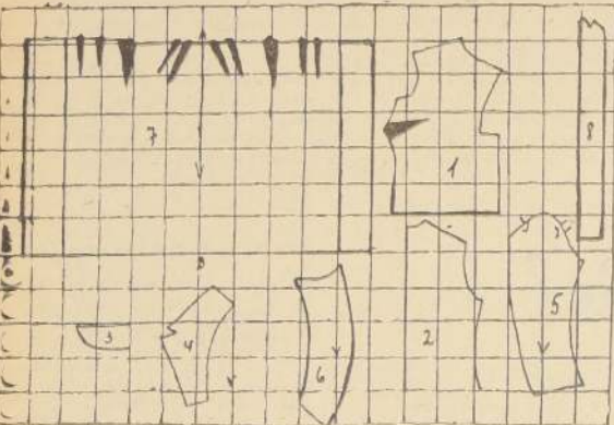
Molde a escala de 10 cm. para talla 44 del traje presentado en Ventana de la Moda. 1.-Mitad delantera. 2.-Mitad espalda. 3.-Parte bajera del cuello. 4.-Cuello mitad. 5.-Parte superior de la manga. 6.-Parte de abajo de la manga.
