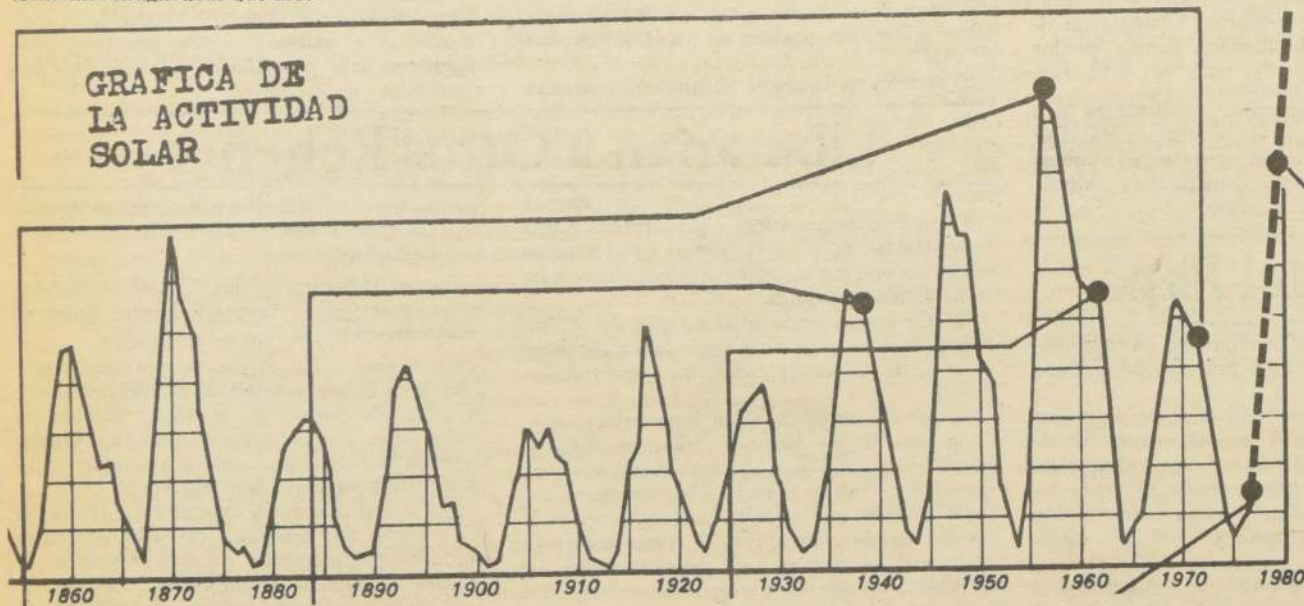
Gráfica de la actividad solar en los últimos cien años.
