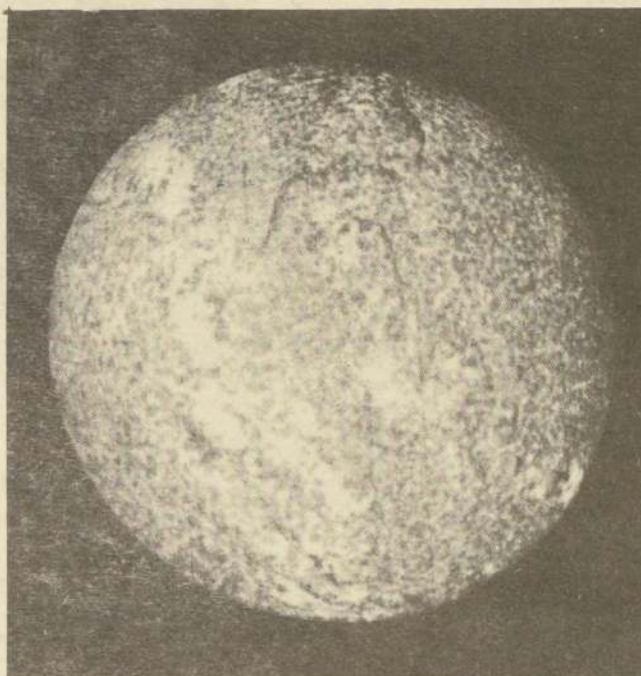
Fotografía del Sol captada con filtro. Pueden observarse las "manchas", verdaderos "bolsones" de magnetismo.
