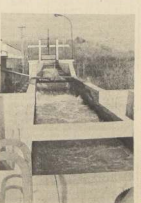
La Empresa Metropolitana de Obras Sanitarias iniciará a fines de año la ampliación de las plantas de agua potable. En la fotografía, un aspecto del departamento de purificación de agua en la Planta de Las Vizcachas.
