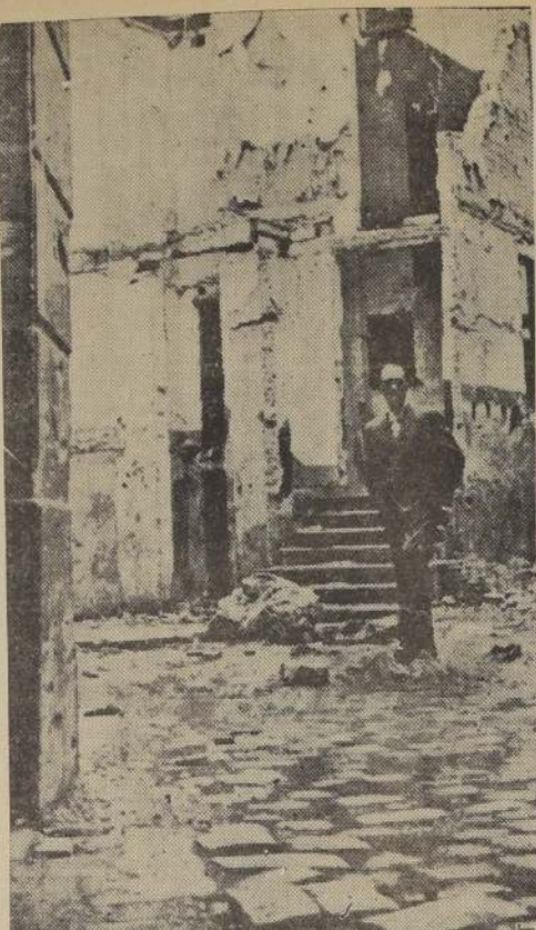
Lorenzo Dominguez, en la Plaza de los Capellanes, en Barcelona, que fué totalmente destruida por una sola bomba fascista que causó 200 víctimas.
