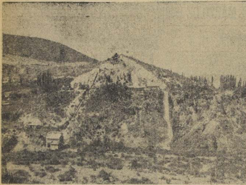
VISTA PANORAMICA DE LA PLANTA HIDRAULICA.— CAPACIDAD, 5,500 H. P.— ALTURA DE CAIDA, 98 METROS.
