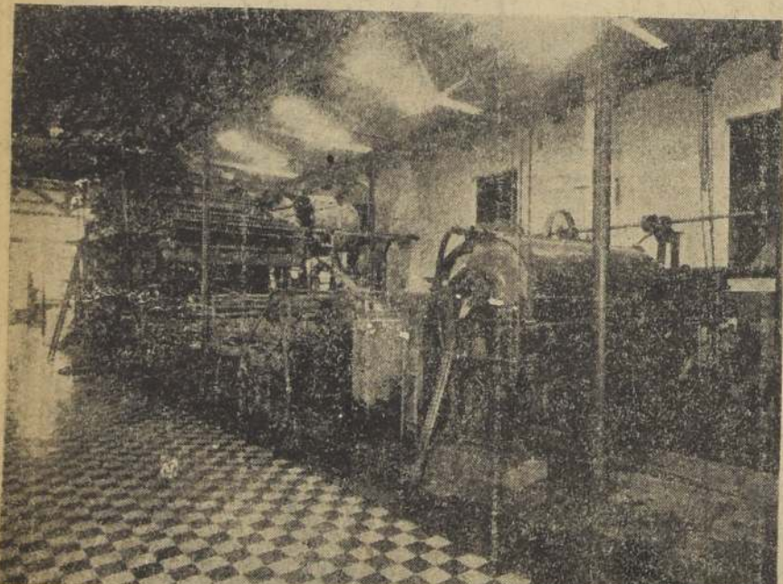
MAQUINA PAPELERA ADQUIRIDA EN 1925.— CAPACIDAD, 10,000 KILOS AL DIA DE PAPELES PARA ENVOLVER.
