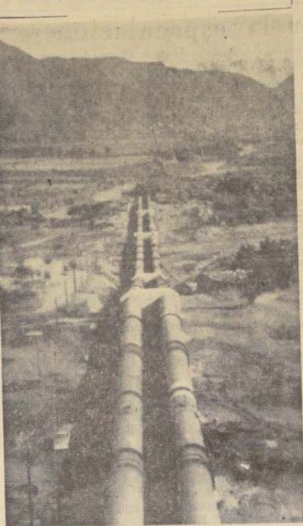
La nueva Central Eléctrica Isla, ubicada en la provincia de Talca, está en su etapa final de construcción. En el grabado, las dos tuberías de acero que llevan el agua hasta las turbinas, se extienden a lo largo de 950 metros, fueron diseñadas y calculadas por ingenieros chilenos, construidas en Huachipato e instaladas por el personal técnico de ENDESA.
