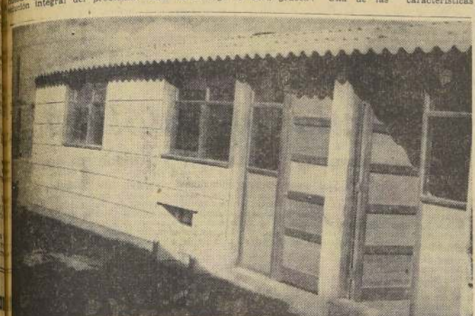
Detalle de una de las casas construidas con el sistema Hellenit. Consta de living-comedor, cocina, baño y dos dormitorios. La cocina tiene salida independiente por la parte de atrás. Los arcos asociados, señores Julio Mardones, Gonzalo Mardones, Sergio González y Jorge Poblete fueron los autores de los planos. Esta casa se encuentra en la Población Dávila, y forma parte de un grupo experimental de cuatro.
