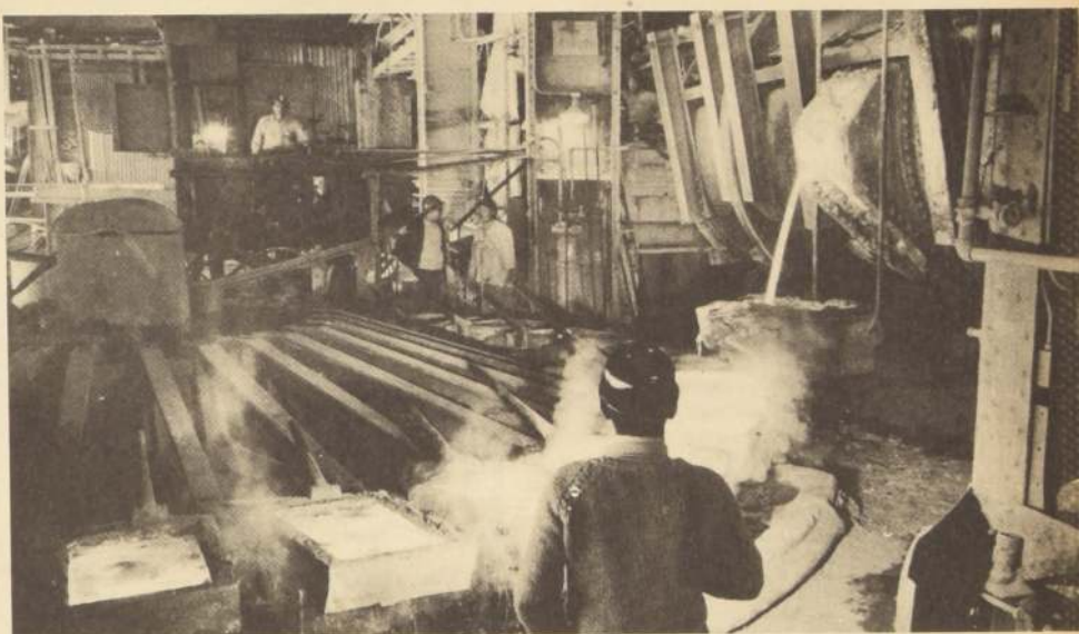
CALETONES. El cobre blister fundido entra a los moldes en la fundición de Caletones de la Sociedad Minera El Teniente.
