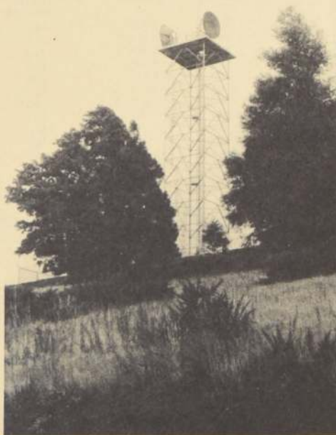
TÍPICAS antenas de Microondas en la Red Troncal Nacional, en Pailahueque y en Mariposas.
