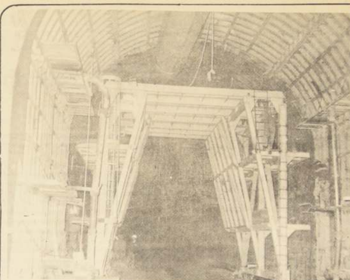
LA PRESIÓN que ejerce el cerro sobre las estructuras del Túnel Lo Prado es posible medirla con el osciloscopio, el que también determina la calidad del material empleado.
