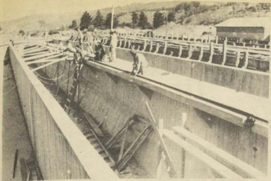
Etapa final de la construcción de los estanques-filtros en la bocatoma del río Maule, de la Planta de Agua de la Industria de Celulosa de Constitución, unidos por un acueducto a las dependencias de la Planta Industrial.
