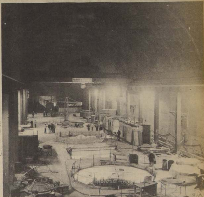
Caverna de la Casa de Máquinas de la Central "El Toro", de 400.000, obra de ENDESA.
