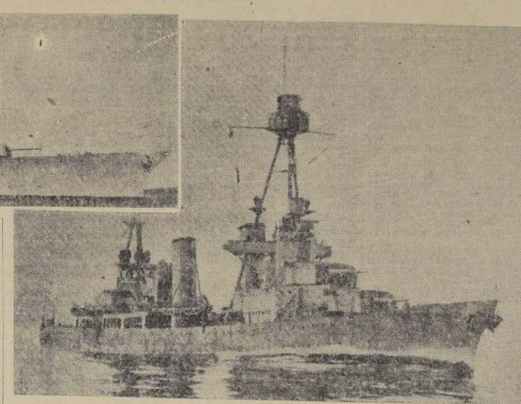
A la izquierda, el "Salt Lake City", gemelo del "Pensacola". A la derecha, el "Houston", a cuya serie también pertenece el "Chester" y el "Chicago". Todas estas modernas naves de guerra cuentan con catapultas para el lanzamiento de los hidroaviones de que van provistas—dos máquinas cada crucero.
