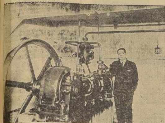
MAQUINA COMPRESORA BORSIG, DE 25.000 FRIGORIAS Y QUE PERMITE ENFRIAR LA LECHE A TEMPERATURAS BAJO CERO Y QUE A LA VEZ PROPORCIONA EL FRIO NECESARIO PARA LAS CAMARAS FRIGORIFICAS.
