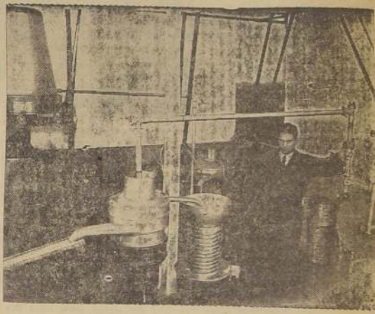
VISTA DE UNA SECCION CON EL PASTEURIZADOR AL FONDO, DESCREMADORA ALFA LAVAL Y ANTI-CALENTADOR
