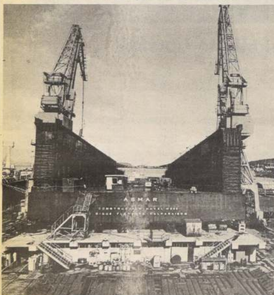
Dique flotante Valparaiso III en grada de construcción (Talcahuano).
