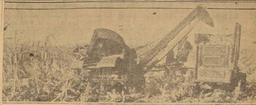
Arrancadora-deshojadora que funciona actuada por un tractor de acoplamiento directo, el cual también tira del carro cargado de espigas. Dos hombres solamente pueden recoger de 4 a 5 hectáreas de maiz por día.
