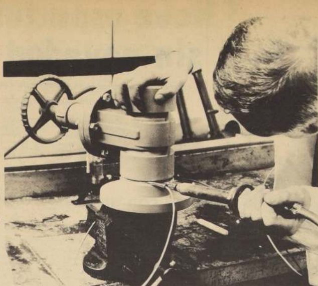
Esta válvula de diafragma totalmente moldeada en polipropileno es soldada a un sistema de irrigación de tubos plásticos.
